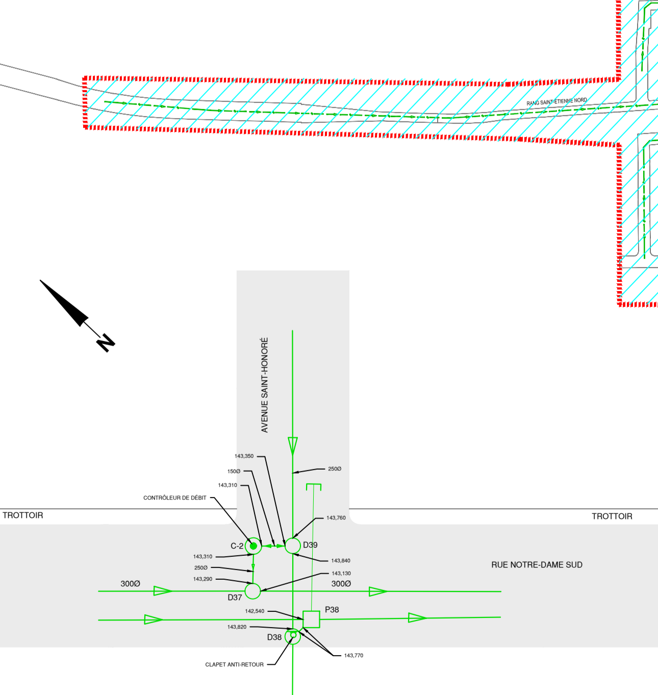
CONTRÔLEUR DE DÉBIT C-2 ÉCHELLE: AUCUNE
