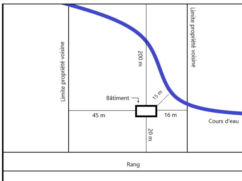
Exemple de plan de localisation
